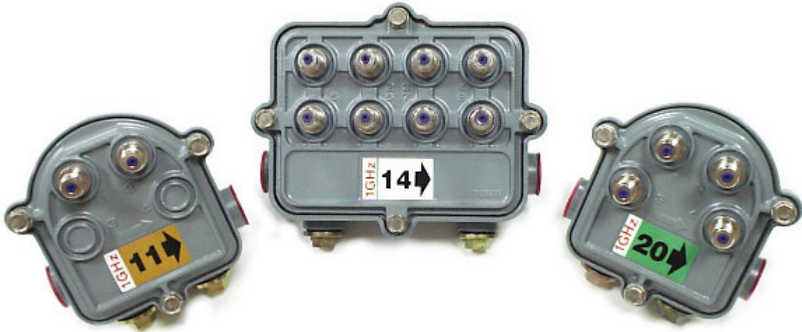
DT55G-SR-200 Series 二路分歧器
